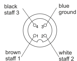
M12 plug
